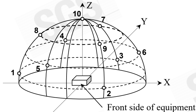
附圖 1. 量測表面的麥克風位置
