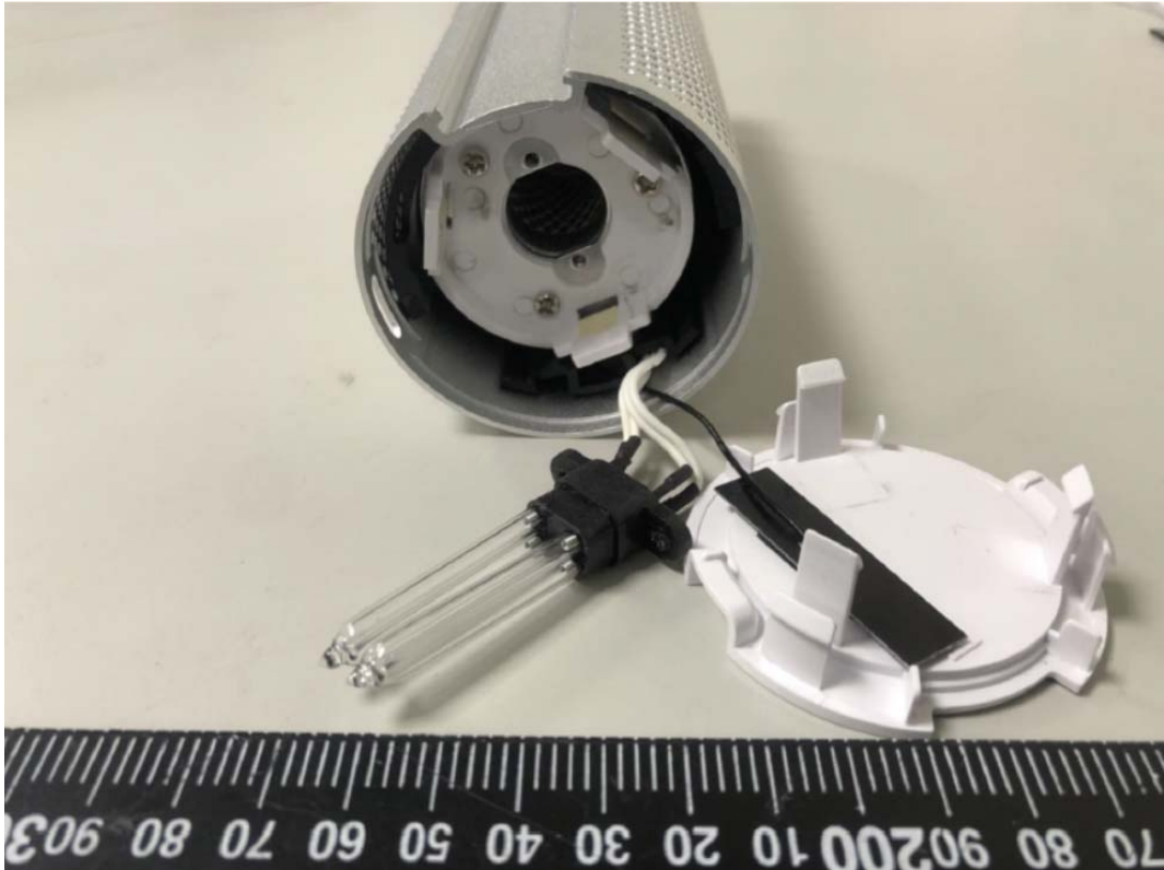
UV Lamp(Type:YLZ04-05)
